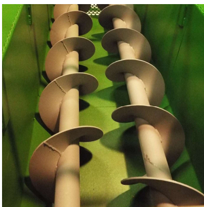
Detalle de sinfín doble
